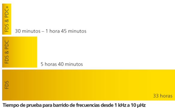
Figura 7: Tiempo de prueba para barrido de frecuencias desde 1 kHz a 10 μHz
