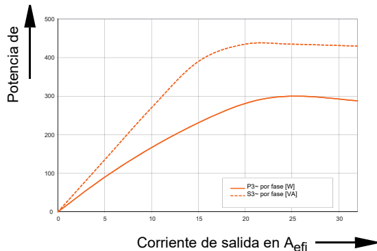
Potencia de salida garantizada por fase de un grupo (los valores de potencia activa en W están garantizados; los valores de potencia aparente en VA son valores típicos)
