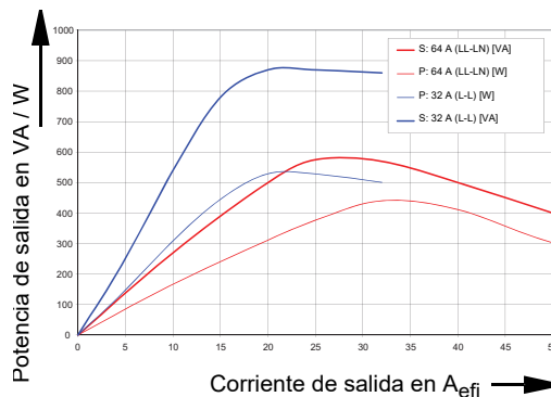
Curvas de potencia de salida monofásica garantizadas (los valores de potencia activa en W están garantizados; los valores de potencia aparente en VA son valores típicos)
