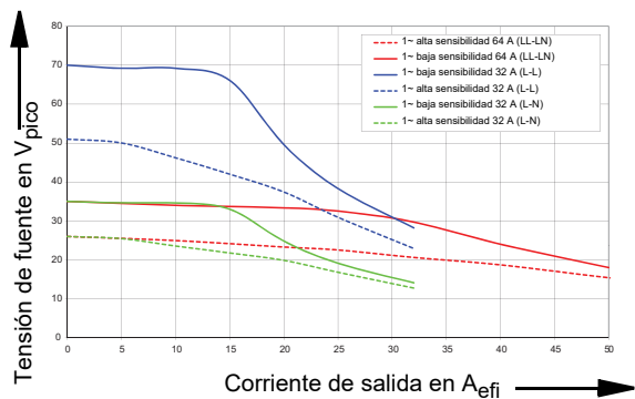
Tensión de fuente típica (50/60 Hz)
