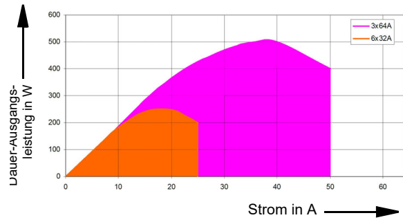
Typ. Dauer-Ausgangsleistung in Abhängigkeit des Ausgangsstroms bei 23 °C; 3- und 6-phasiger Modus
