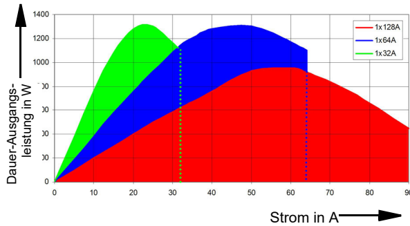
Typ. Dauer-Ausgangsleistung in Abhängigkeit des Ausgangsstroms bei 23 °C; einphasiger Modus
