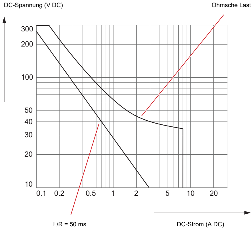
Schaltlast-Grenzkurve der Binärausgangs-Relais für DC-Spannung
