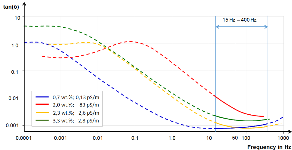
Figura 6. Respuesta dieléctrica de banda ancha de 4 transformadores de potencia diferentes a 20 °C. (Frecuencia en Hz)
