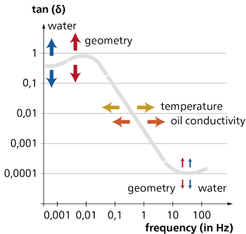
Figura 2. Propiedades dieléctricas del aislamiento de papel-aceite entre el devanado de alta y el de baja tensión de un transformador de potencia (C HL)
