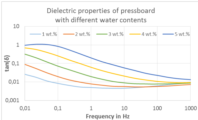
Figura 1. Propiedades dieléctricas del cartón prensado impregnado en aceite con diferentes contenidos de agua a 20 °C. (Propiedades dieléctricas del cartón prensado con diferentes contenidos de agua. Frecuencia en Hz, 1 % en peso)
