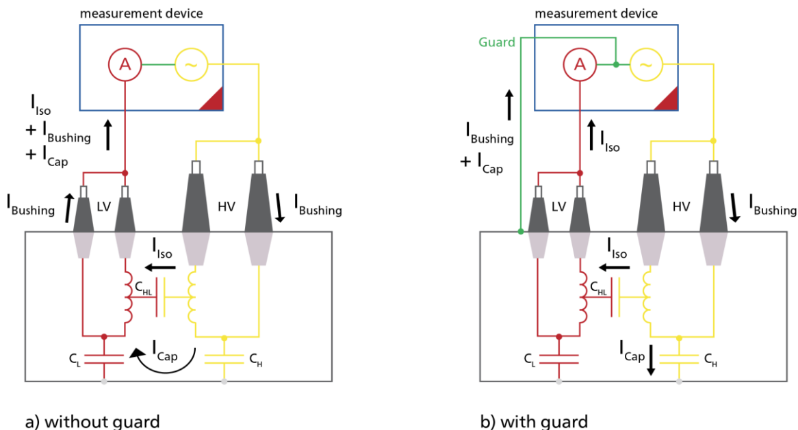
Figura 4. Medición de CHL en un transformador de dos devanados con y sin guarda (dispositivo de medición; ais; borna; Cap; sin guarda; Guarda; con guarda)
