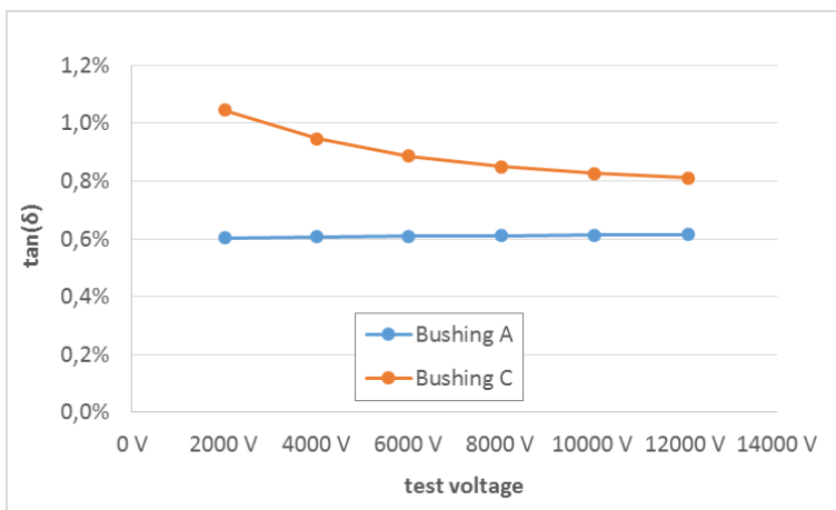
Figura 9. Mediciones de la \tan(\delta) de dos bornas RBP 123 kV del mismo tipo a diferentes tensiones con problemas de contactos en la toma de medición de la borna C (datos de [8]) (Bornas A, Bornas C; tensión de prueba)
