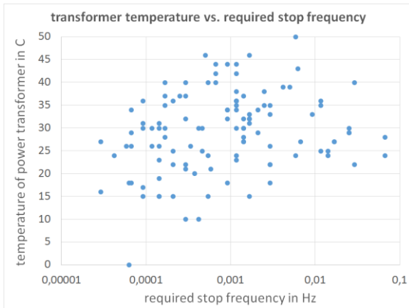
Figura 7. Frecuencia de parada requerida, dependiendo de la temperatura del transformador en un estudio que incluye más de 100 transformadores de potencia (temperatura del transformador frente a frecuencia de parada requerida; temperatura del transformador de potencia en C; frecuencia de parada requerida en Hz)
