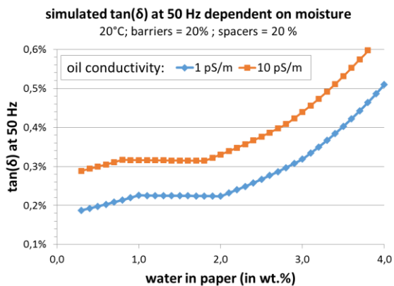
Figura 2. Propiedades dieléctricas del aislamiento de papel-aceite entre el devanado de alta y el de baja tensión de un transformador de potencia (C HL)
