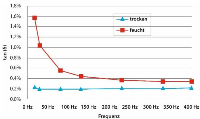
Abbildung 1: Verlustfaktor in Abhängigkeit von der Frequenz bei einer trockenen und einer feuchten 33 kV-OIP-Durchführung bei 30 °C (Daten aus Invalid source specified.)
