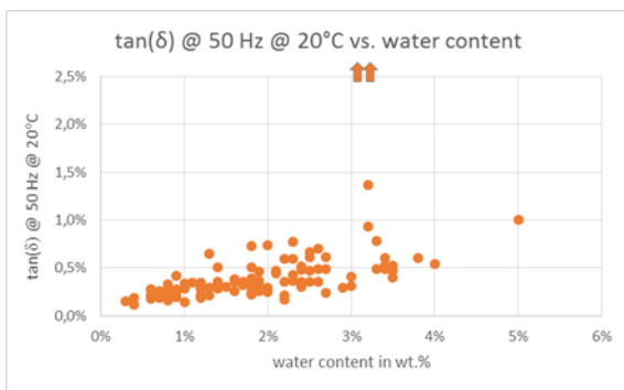
Figura 5. Relación de la \tan(\delta) a 50 Hz y 20 °C con el contenido de agua en la celulosa en más de 100 transformadores de potencia, evaluada a través de medición dieléctrica de banda ancha utilizando el sistema de pruebas DIRANA de OMICRON. ( \tan(\delta) a 50 Hz a 20 °C y contenido de agua; contenido de agua en % en peso)
